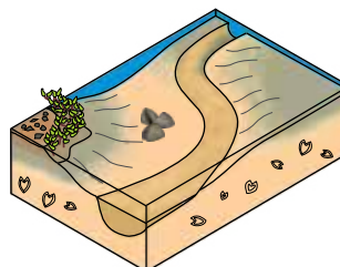
Dachsteinski apnec se je odlagal na plitvem morskem dnu. Značilno je menjavanje gostega apnenca, breče in stromatolitov.
