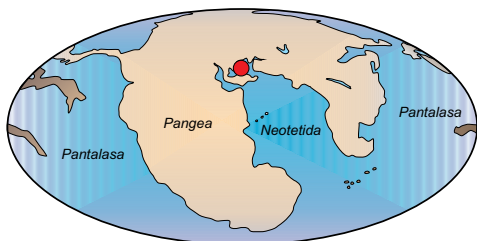
Podoba sveta v času mlajšega triasa. Položaj morskega dna, na katerem se je odlagal apnec, ki danes najdemo v kamnolomu Ušenišče, je označen s piko. Prerejeno po Chablais in soavtorji (2011).
